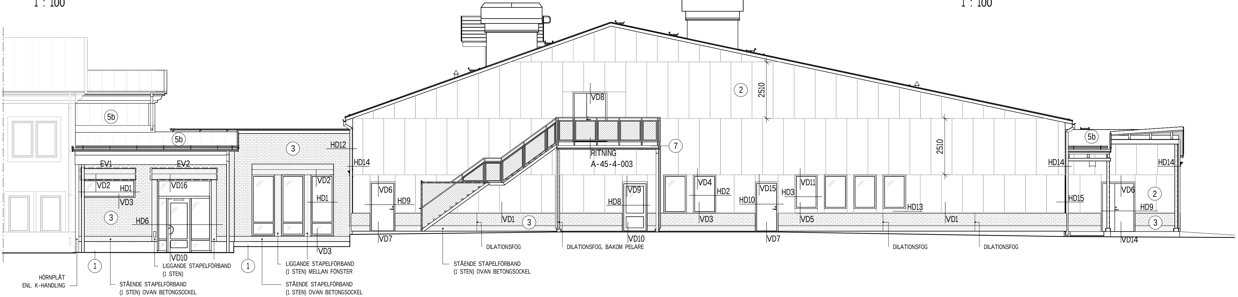
FASAD MOT NORDÖST 1 : 100
