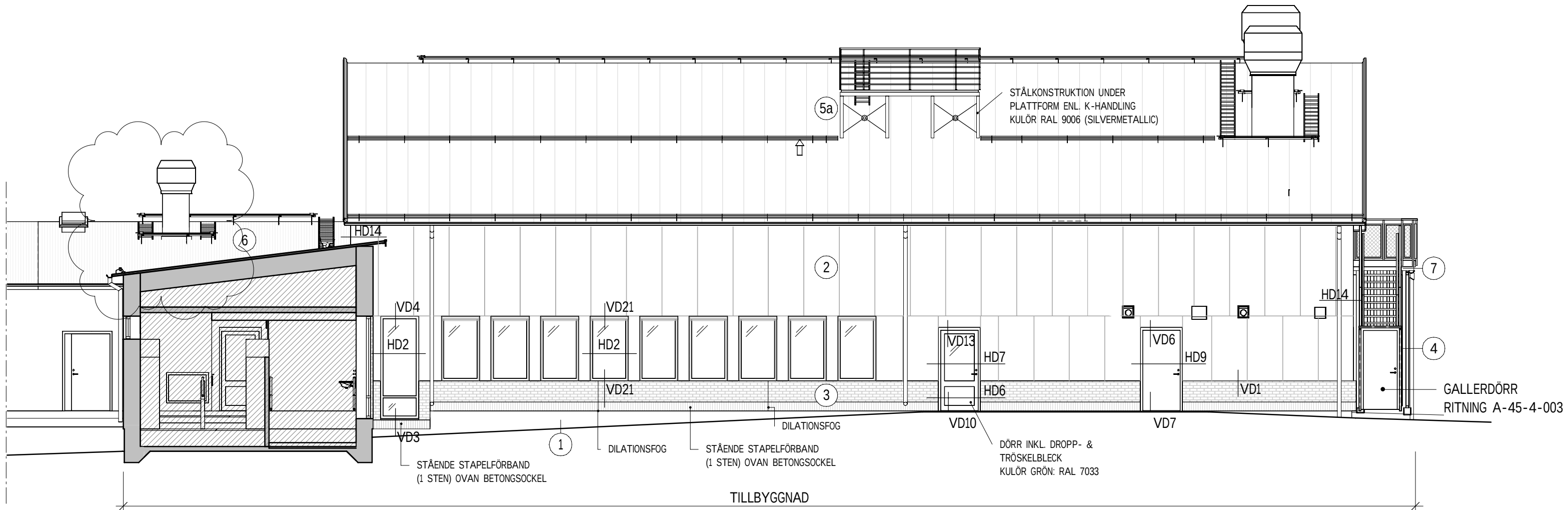
FASAD MOT SYDÖST 1 : 100
